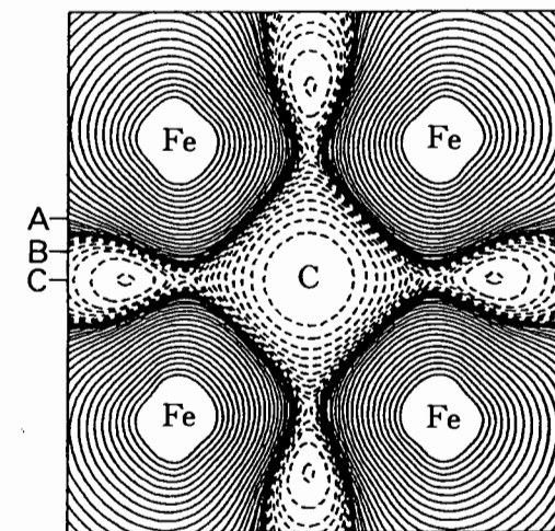
鉄中炭素のスピン密度
